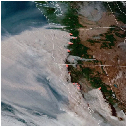
Una imagen del satélite GOES-17 de la NOAA del 8 de septiembre de 2020 que muestra la presencia del humo y el calor de los incendios forestales del oeste de EE. UU.
